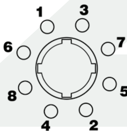
Grafik 12-2 - Acht Bolzen
