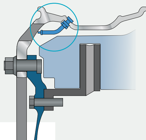
Grafik 4-2 Innenventil
